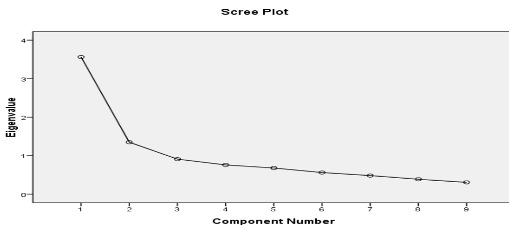
شکل ۱- منحنی شیب اسکری
