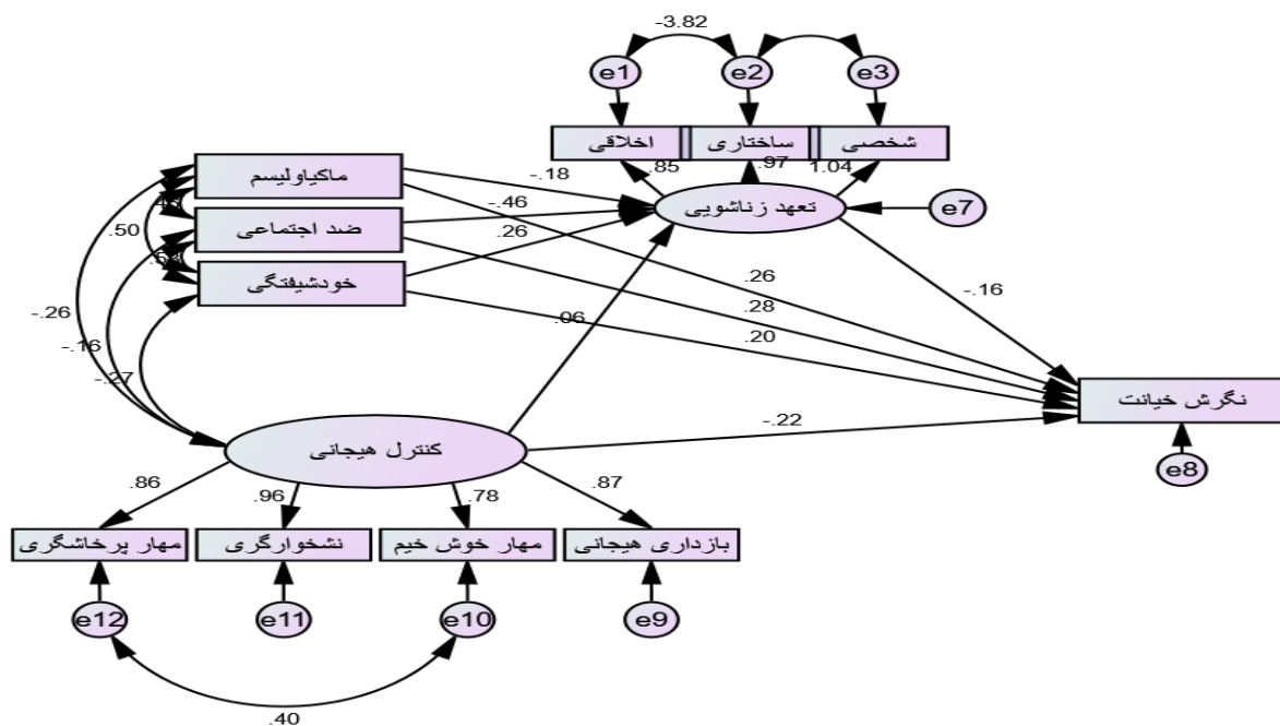
شکل ۱. مدل آزمون شده همراه با ضرایب استاندارد مسیرها
