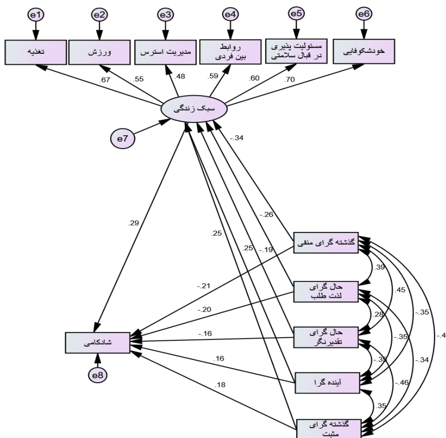
شکل ۱: ضرایب مسیر در حالت استاندارد
