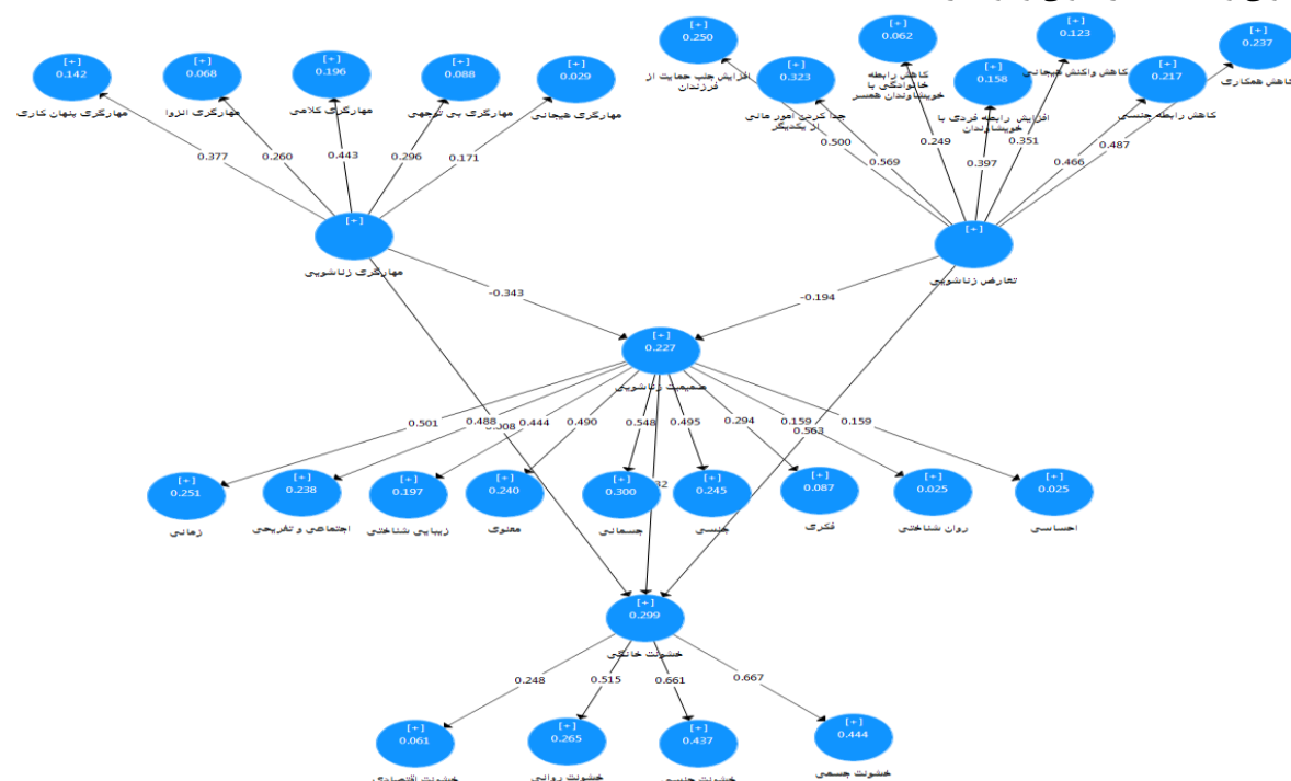
شکل ۱، نمودار مسیر ضرایب استاندارد در مدل
