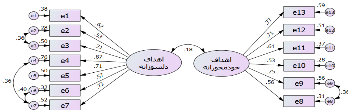
شکل ۱. مدل تحلیل عاملی تأییدی با ضرایب استاندارد شده
