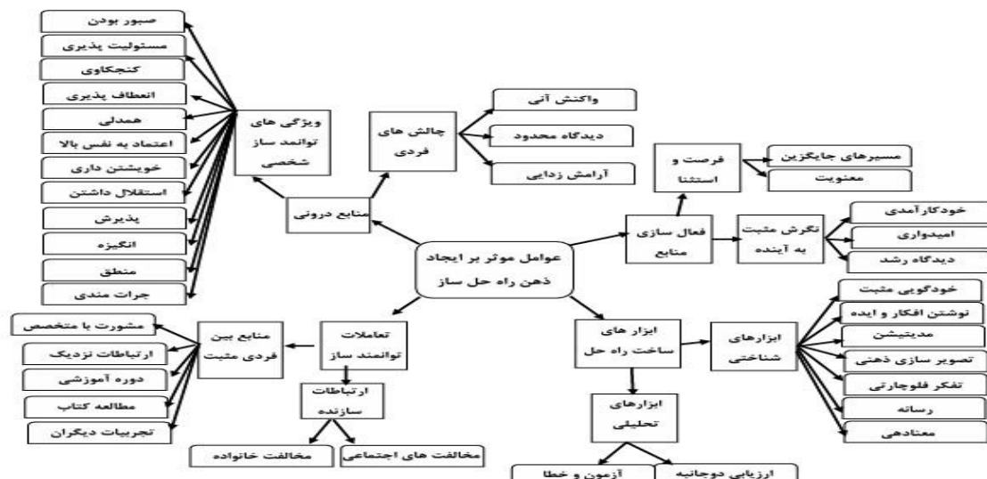
شکل ۱. مدل مفهومی عوامل مؤثر بر ایجاد ذهن راه حل ساز
